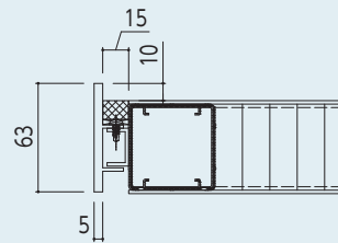
幕板B
