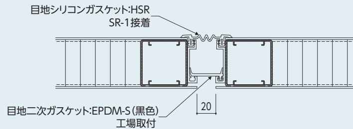
50Hタイプ断面
