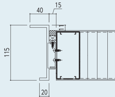
幕板A
