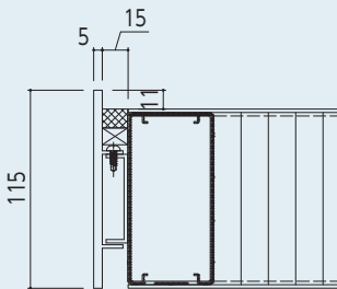
幕板B
