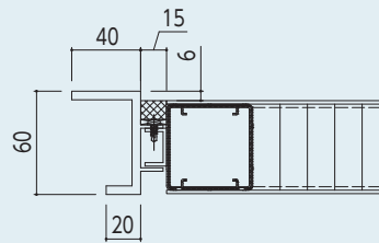
幕板A
