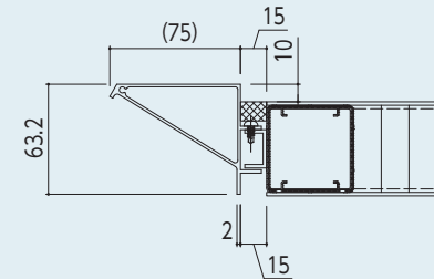
鼻先
