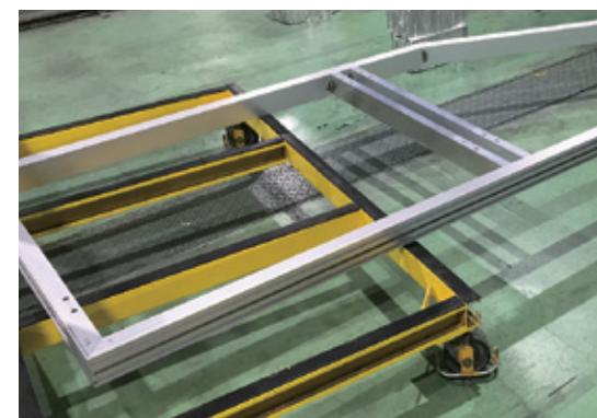
枠組
