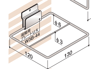
シューズフックD W3B-25 クロームメッキ 梱包入数 30
