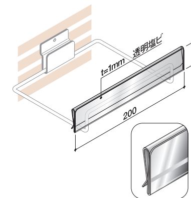
ボックスホルダー W3B-31 クロームメッキ 梱包入数 100
