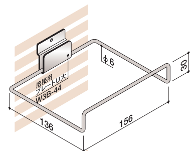
FU型シューズフック W3B-22 クロームメッキ 梱包入数 30
